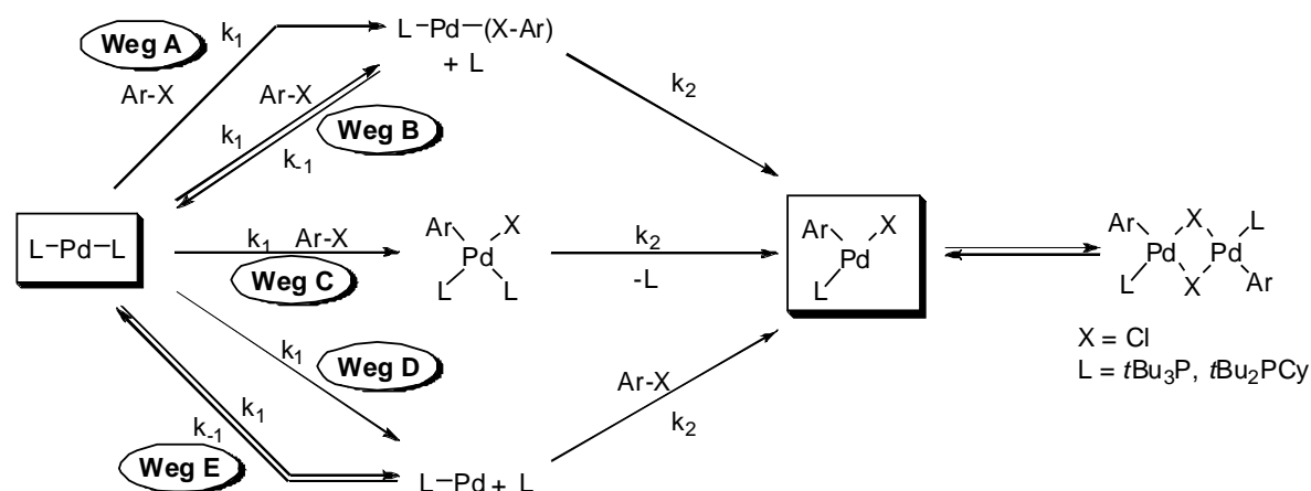
Abbildung 5: Mögliche Mechanismen der oxidativen Addition von Ar-X.
