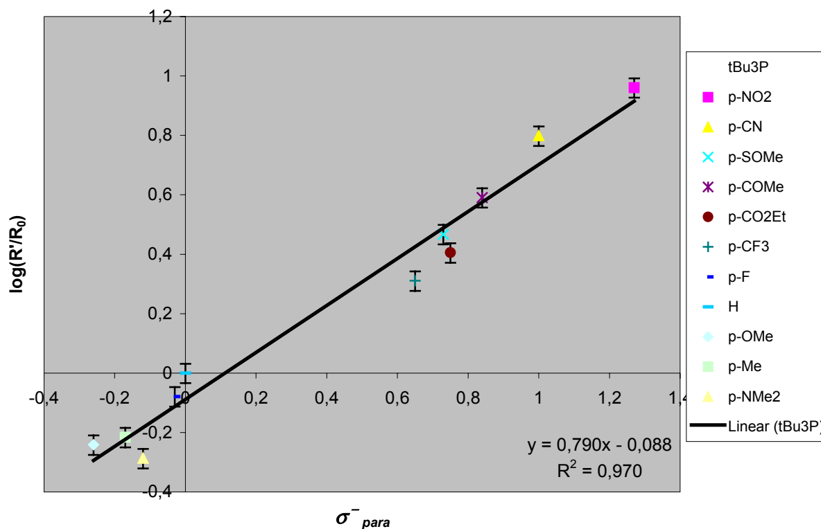
Abbildung 111: Hammett-Auftragung der Ergebnisse aus dem Screen für die para -Bromaromaten unter der Annahme eines negativen Übergangszustands. Es wird das Phosphin tBu 3 P P 18 bei einem Komponentenverhältnis von Pd/Cu/PR 3 4:3:4 eingesetzt.
