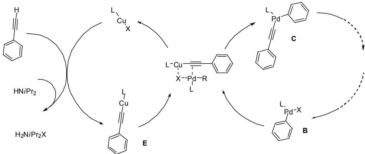
Abbildung 100: Korrigierte Darstellung des Acetylen-Aktivierungszyklus von Cu(I).
