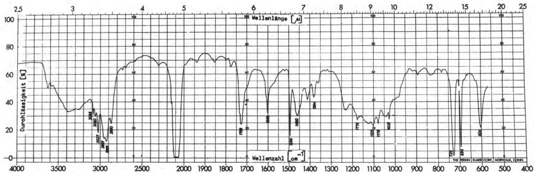
Abb. 10 Tiefdruckfarbe (Blau B), flüssig, Schichtdicke 0,015 mm in einer Flüssigkeitsküvette mit KBr-Fenster
