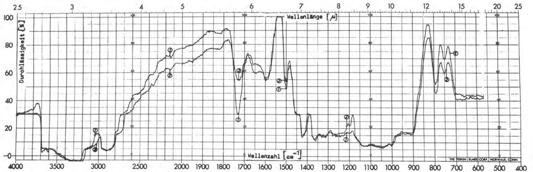
Abb. 2 Zwei verschiedene Tiefdruckpapiere, fest, Flächengewicht für beide 60 g/m 2 (Beide Spektren sind mit ca. 13-facher Ordinatenrückdehnung aufgenommen)
