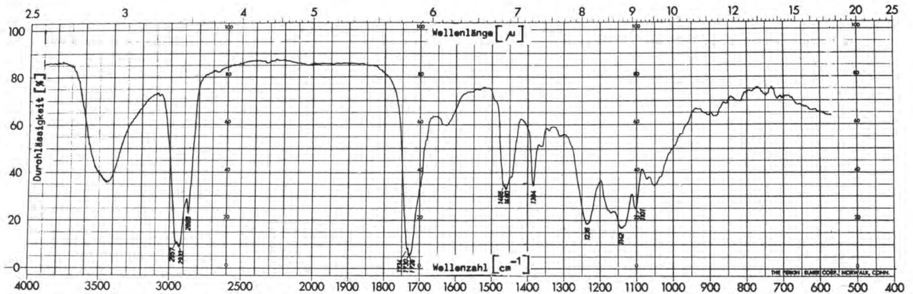
Abb. 14 Kolophoniumharz mit Acrylsäure modifiziert, fest, 1 mg in 13 mm \Phi Preßling mit 200 mg KBr
