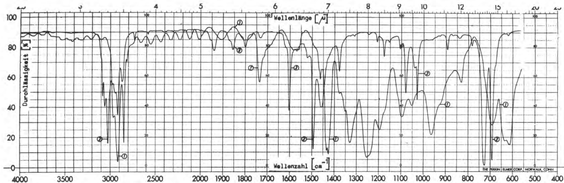
Abb. 5 Kurve 1, Hart PVC-Folie Genotherm, fest, Folienstärke ca. 0,040 mm Kurve 2, Toluol, flüssig, Schichtstärke 0,017 mm in einer Flüssigkeitsküvette mit KBr-Fenster
