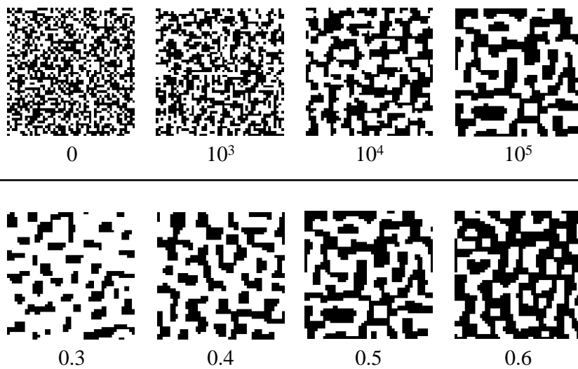
Abbildung 6.8: Obere Reihe: Umbesetzung der besetzten Gitterplätze (schwarze Punkte) mit ansteigender Zahl von Umbesetzungen (Angabe unter dem jeweiligen Bild). Die Bedeckung wurde zu 0.5 gewählt, die Größe des Gitters beträgt 50 \times 50 . Untere Reihe: Laterale Verteilung der besetzten Gitterplätze nach der Umbesetzung ( 10^5 Umbesetzungen) für verschiedene Besetzungen (Angabe unter dem jeweiligen Bild). Die Größe des Gitters beträgt wiederum 50 \times 50 .
