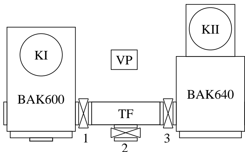
Abbildung 3.6: Prinzipskizze des Vakuumsystems mit den beiden Vakuumkanern (BAK 640 und BAK 600) und des Transfersystems (TF). Bezeichnungen: Kryopumpen (KI, KII), Vorpumpe (VP), Schnittstellen zum Transfersystem (1-3). Die Verbindungen der Vorpumpe zu den Kamern wurde aus Gründen der Übersichtlichkeit nicht eingezeichnet.
