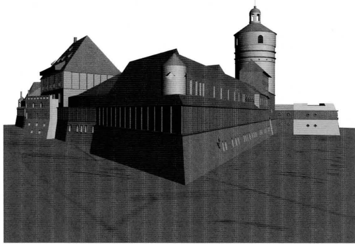
Abb. 21. Leipzig, Pleißenburg um 1600. Schematische CAD-Rekonstruktion.
