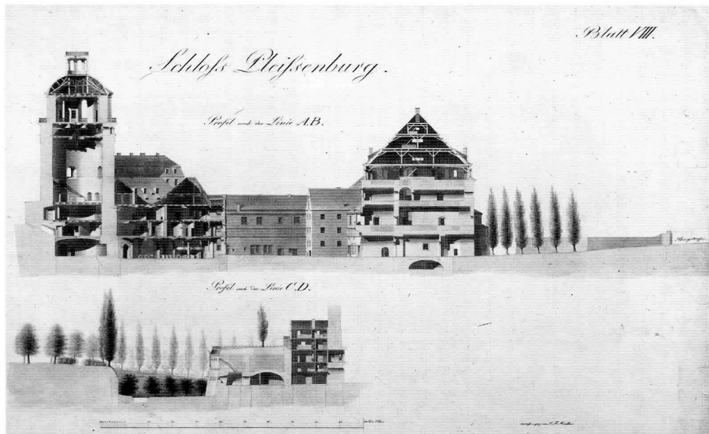
Abb. 20. Schnitt durch die Pleißenburg um 1827.
