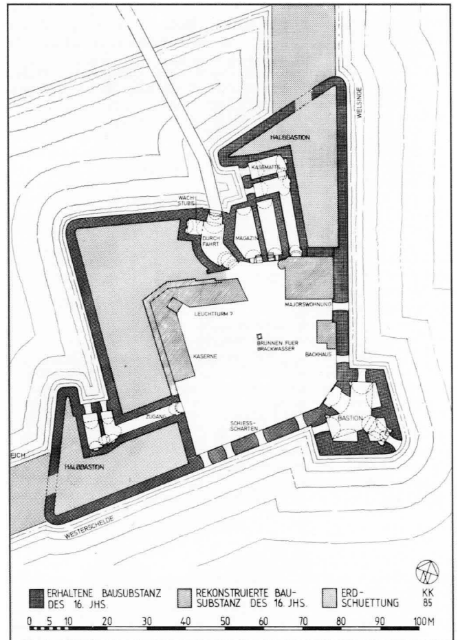
Abb. 17. Fort Rammekens. Rekonstruierter Grundriss der Festung von 1547. Nach Kiem (Anm. 80, 1987) Abb. 2.
