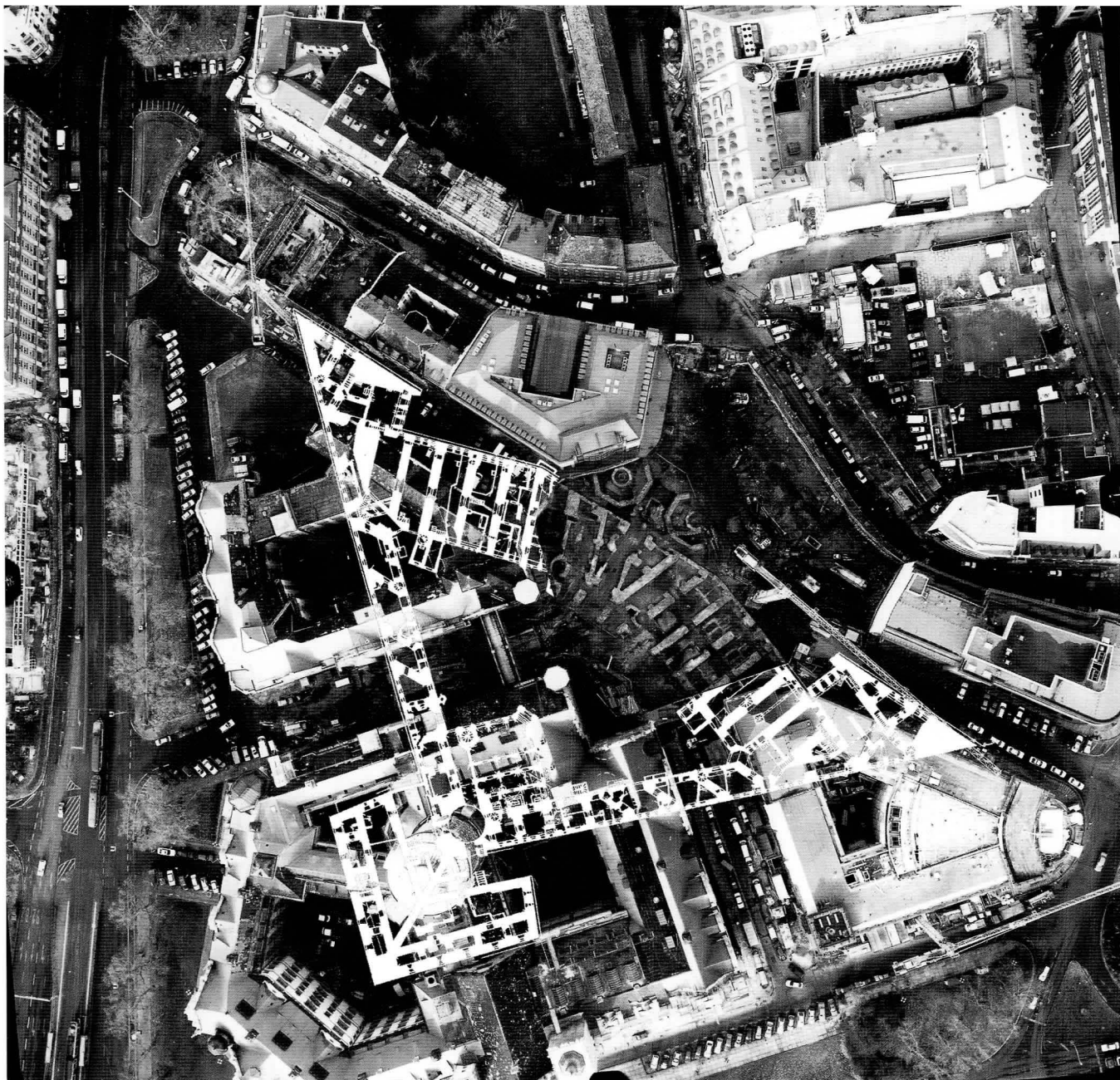
Abb. 26. Leipzig. Luftbild mit eingeblendetem Grundriss der Pleißenburg (Messflug Dez. 1995). Ingenieurbüro für Luftbilddauswertung und Vermessung – Borna.
