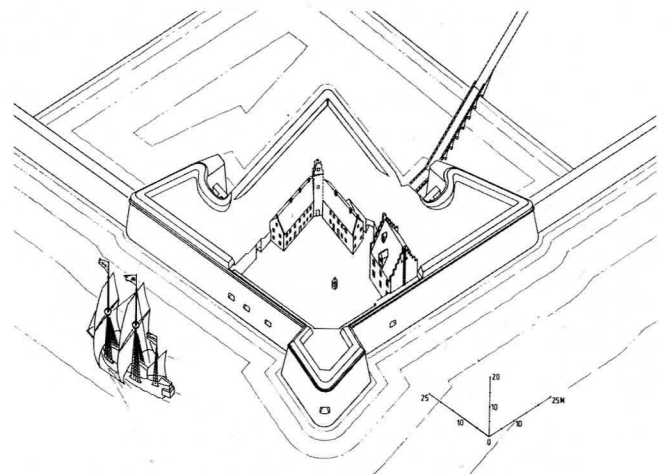
Abb. 18. Fort Rammekens. Isometrie der rekonstruierten Festung von 1547. Nach Kiem (Anm. 80, 1987) Abb. 5.
