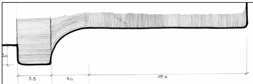
102. Rahmung / Schnitt mit angedeuteter Sandsteinscharrierung
