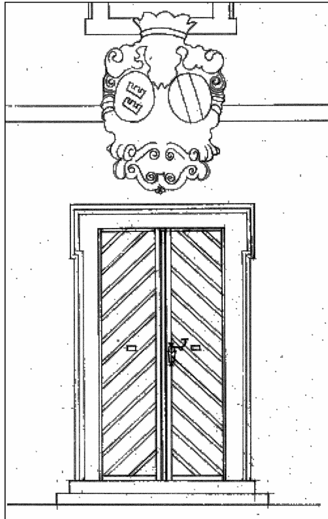
101. Zeichnung Eingangsportal nach Aufmass
