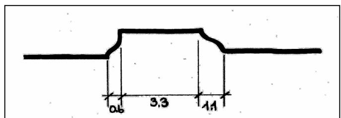
103c. Profilierungsdetail A, Türflügel Innenseite
