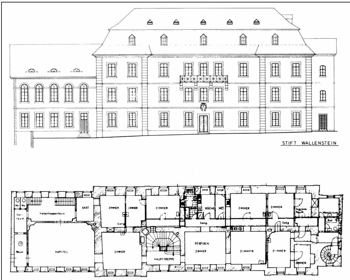
96. Eingangsfassade und Grundriss 1. Obergeschoss
