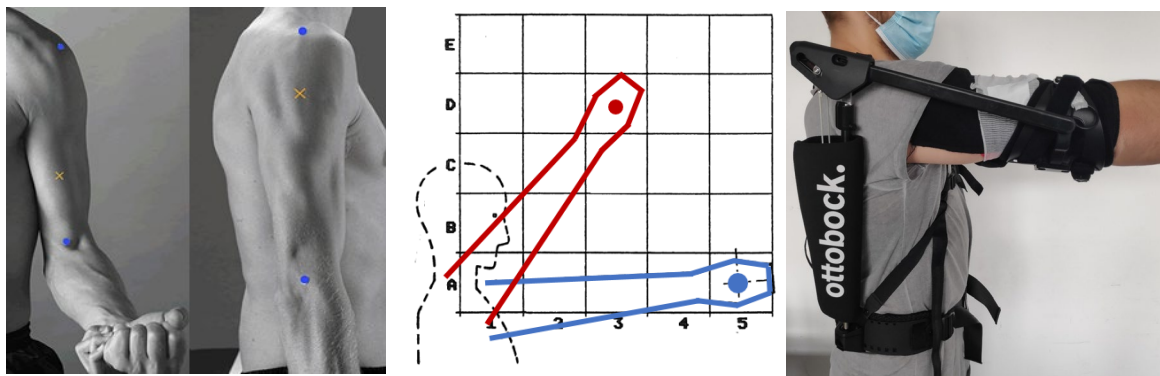
Abbildung 1: Links – Platzierungspunkte des Messgeräts auf M. biceps brachii und M. deltoideus pars acromialis nach SENIAM (2004). Mitte – Armpositionen A5 (blau) und D3 (rot) nach Bier (1991). Rechts – Proband mit PortaMon NIRS und passivem Exoskelett Paexo Shoulder.
