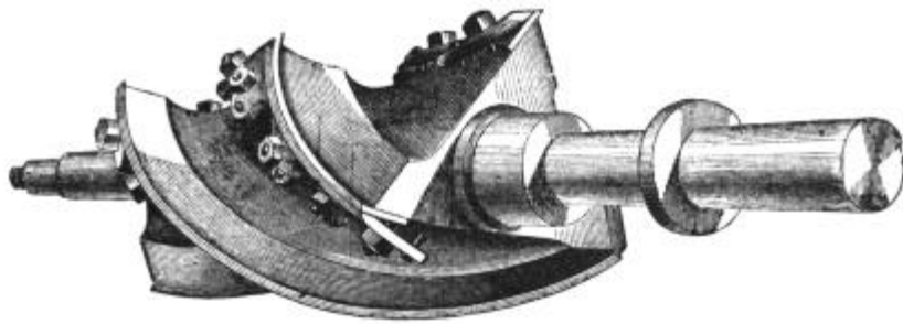
Abbildung 31: Spiralmesserwelle von Marechal & Godeau, ausgeführt von der Firma Arbey, Paris.
