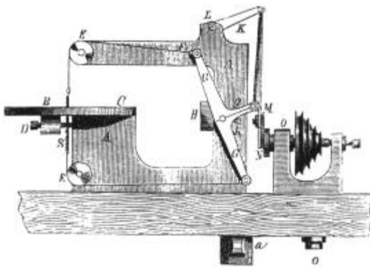
Abbildung 68: Schweifsäge zum Ausschneiden von Verzierungen in Holz, Elfenbein usw.
