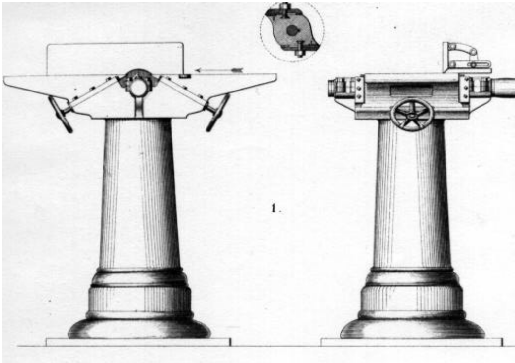
Abbildung 53: Handplaner and Jointer von Fay & Co., Cincinnati, U.S.A. Vorderansicht und Seitenansicht der Maschine sowie Schnitt durch die Messerwelle (Bildmitte).
