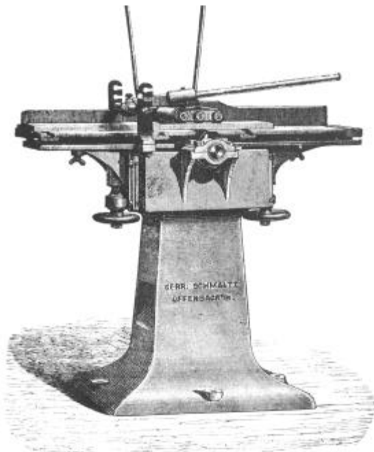
Abbildung 54: Ein mit An- druckwalzen versehenen Abrich- ter der Firma Schmaltz zum Hb- beln längerer Werkstücke. Die Handandruckwalze konnte, je nach der Dicke der Hölzer, ver- schieden hoch eingesetzt werden.
